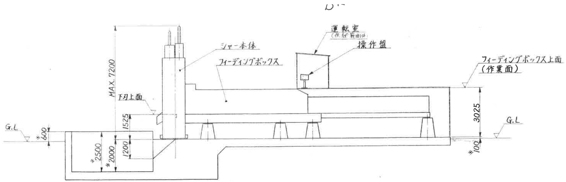
断面図 A-A
