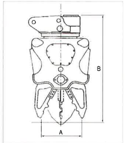
■寸法図
